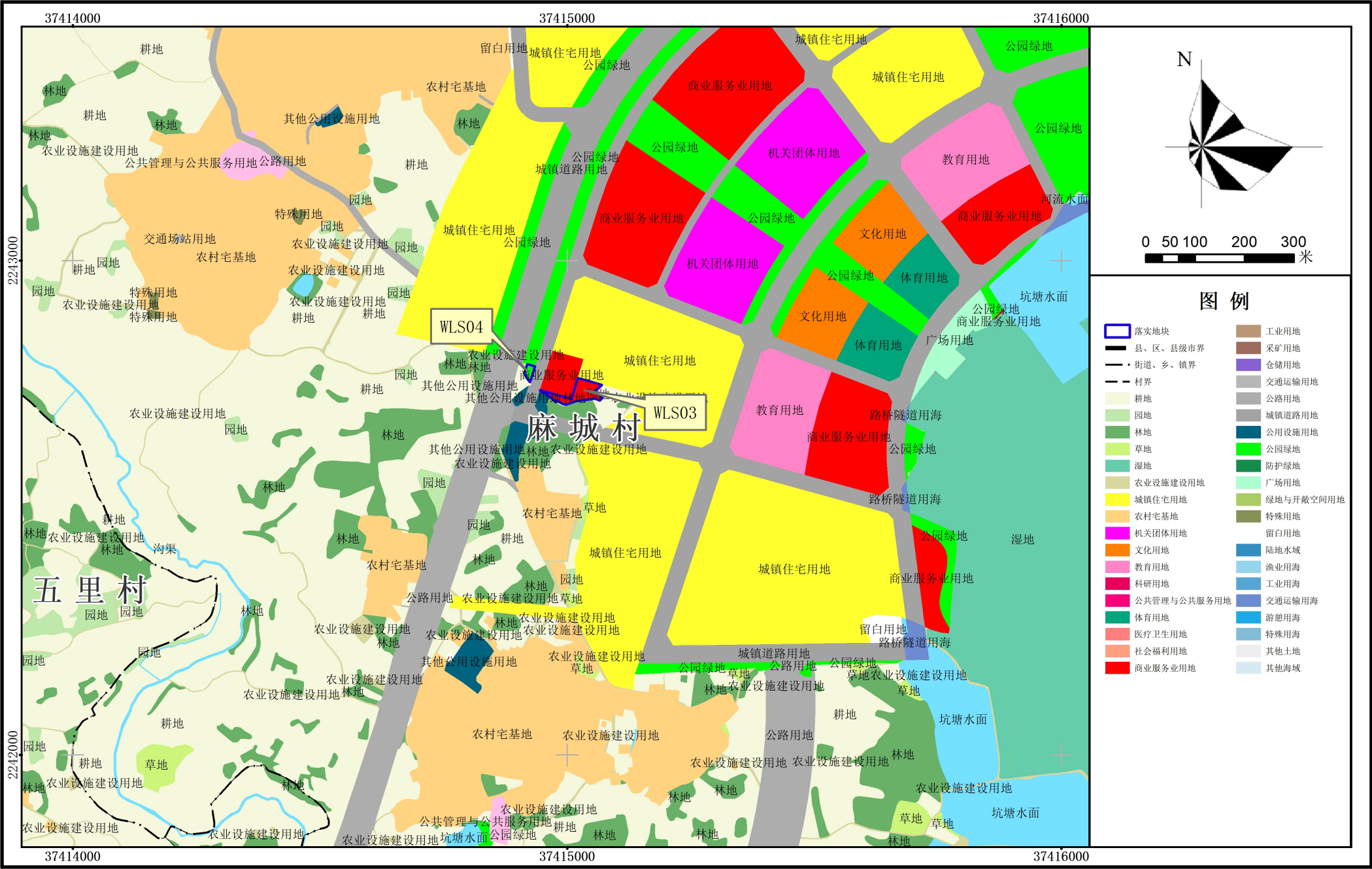
落实后地块土地使用规划图（WLS03、WLS04）
