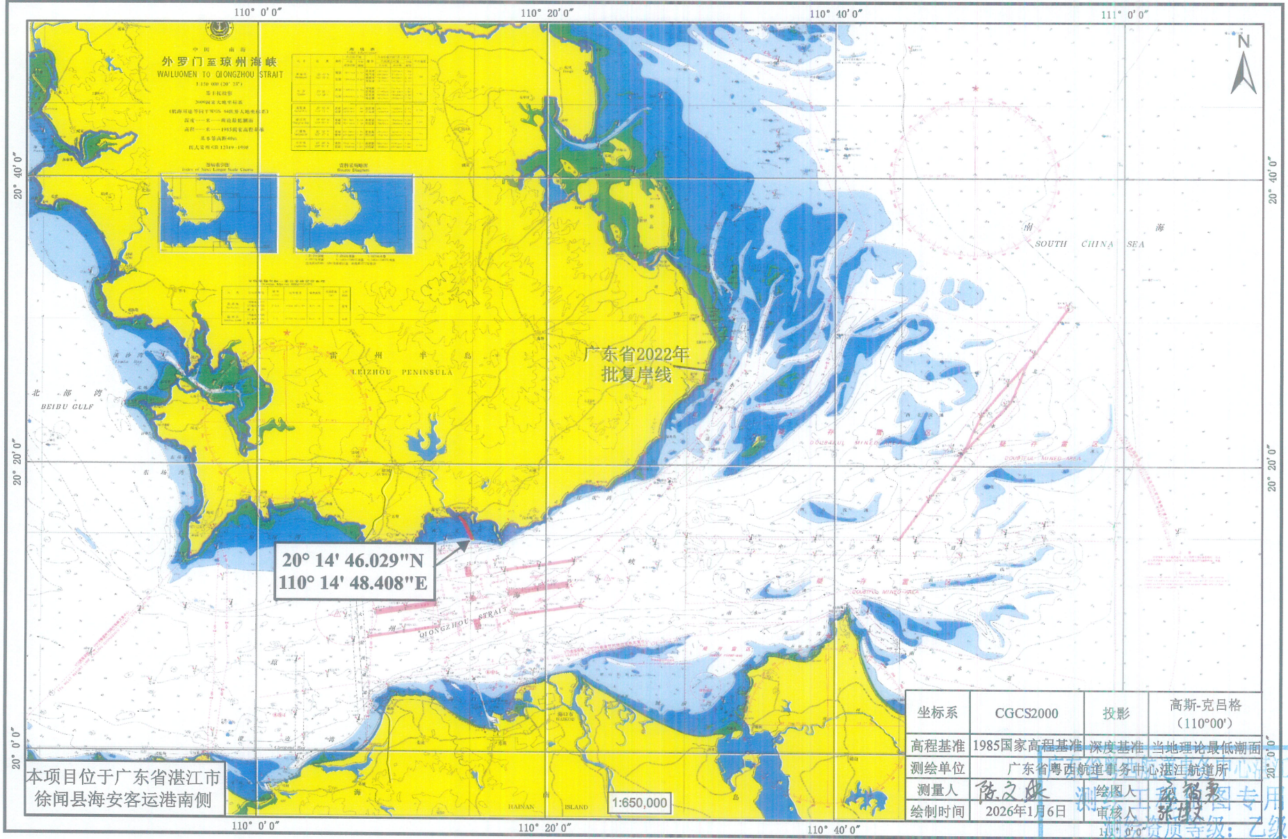
海安（客运港）航道疏浚项目宗海位置图
