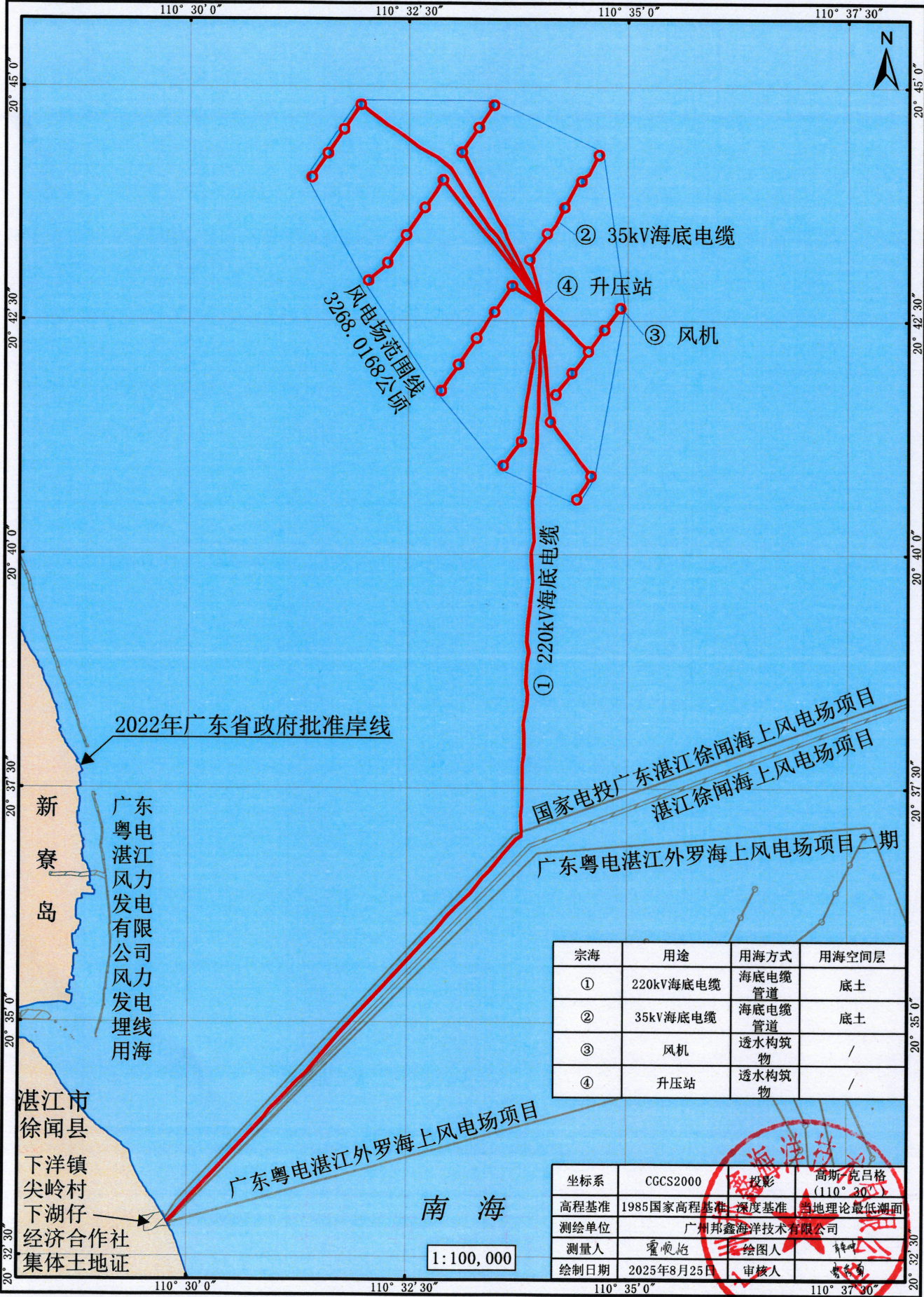
广东粤电湛江新寮海上风电项目宗海平面布置图
