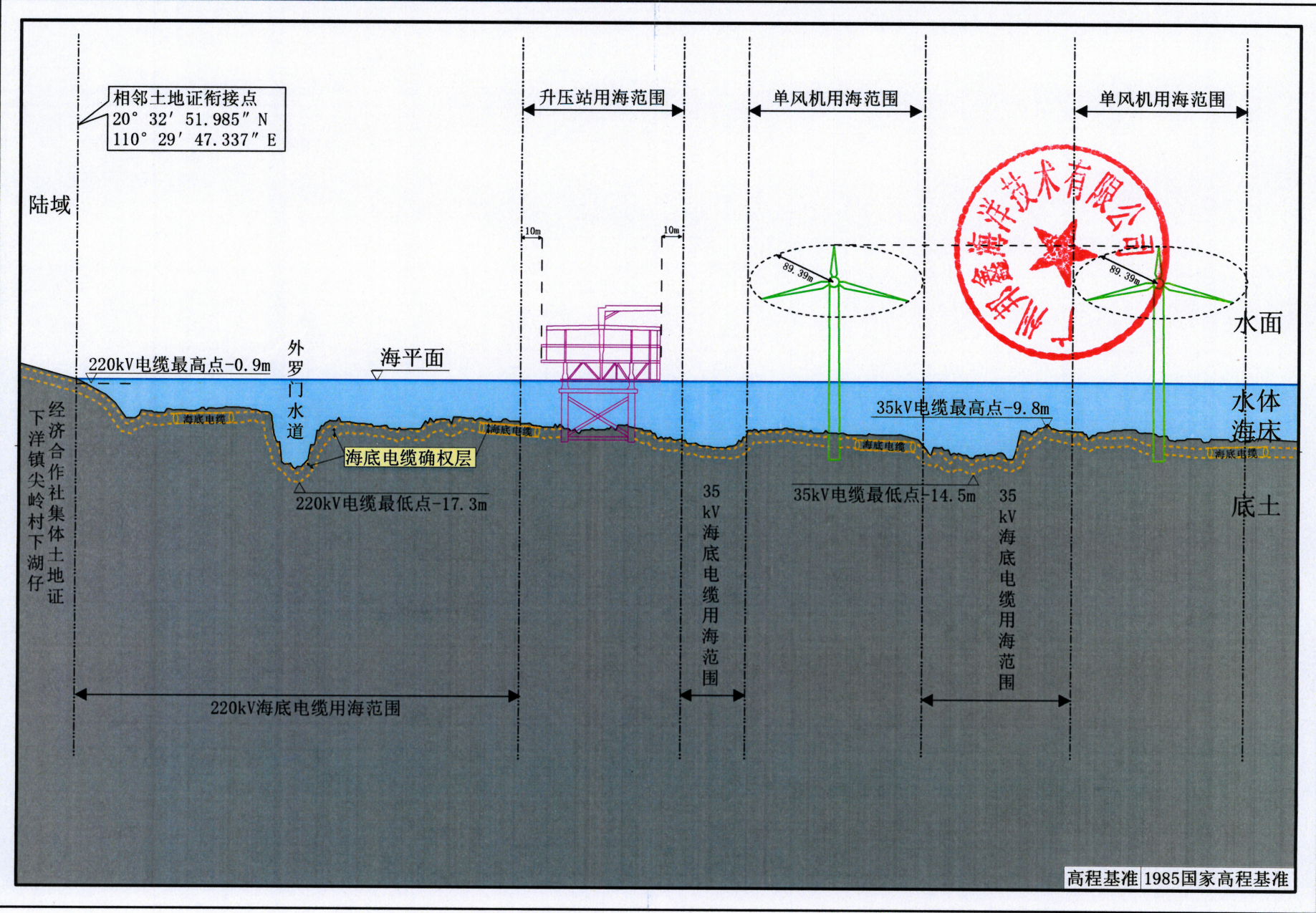
广东粤电新寮海上风电项目宗海立体空间范围示意图
