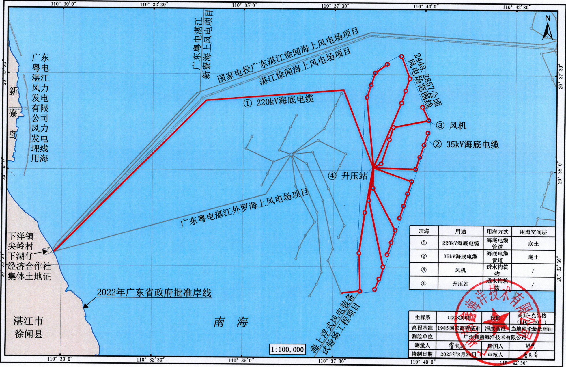
广东粤电湛江外罗海上风电项目二期项目宗海平面布置图
