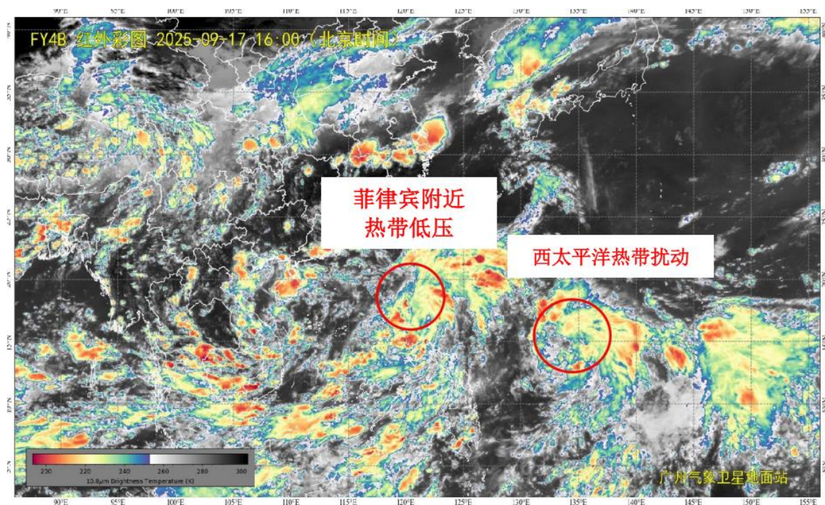
图 1 2025 年 9 月 17 日 16:00 时卫星监测实况
