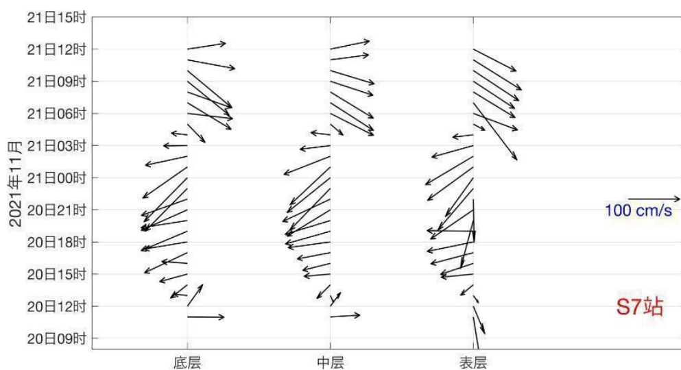
图 3-10g S7 站实测海流矢量图
