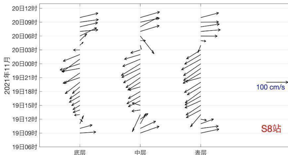
图 3-10h S8 站实测海流矢量图
