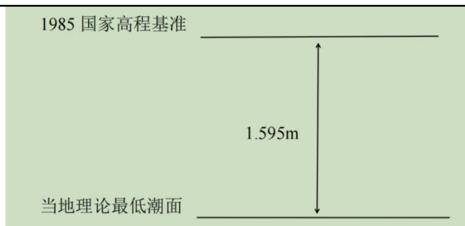
图 3-6 当地基面关系示意图
