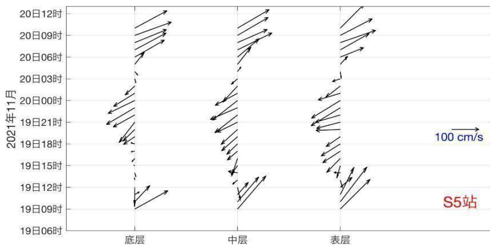
图 3-10e S5 站实测海流矢量图
