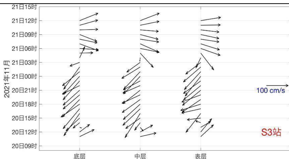
图 3-10c S3 站实测海流矢量图
