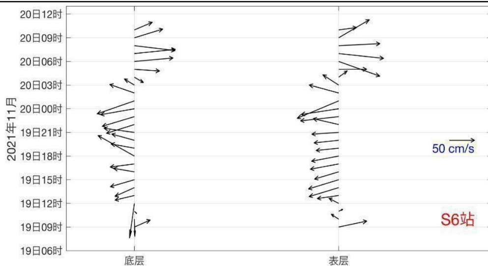
图 3-10f S6 站实测海流矢量图
