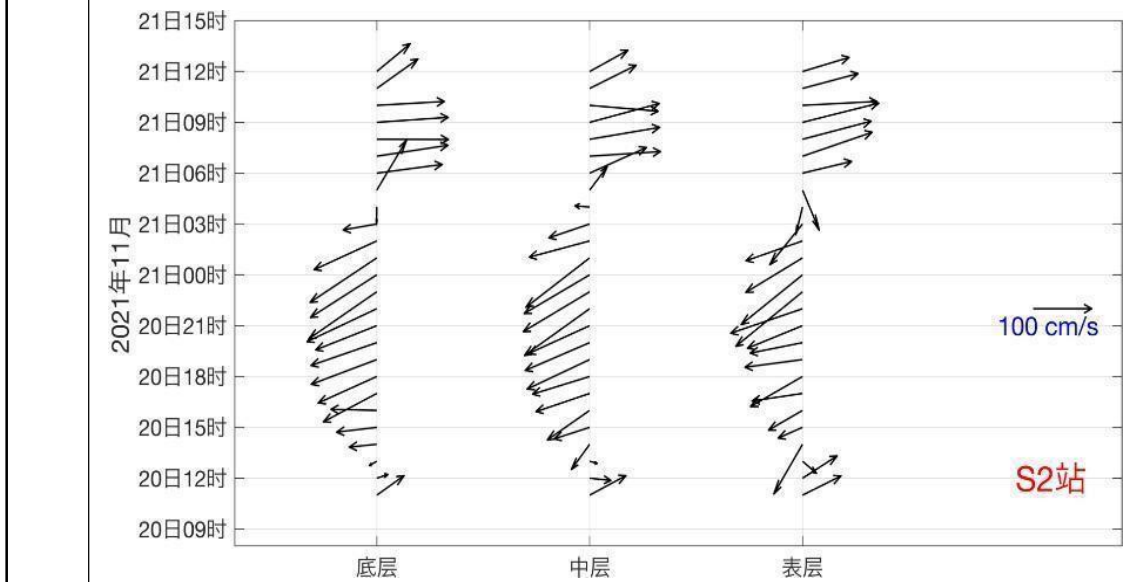
图 3-10b S2 站实测海流矢量图
