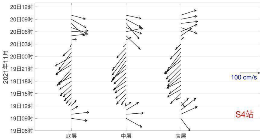
图 3-10d S4 站实测海流矢量图
