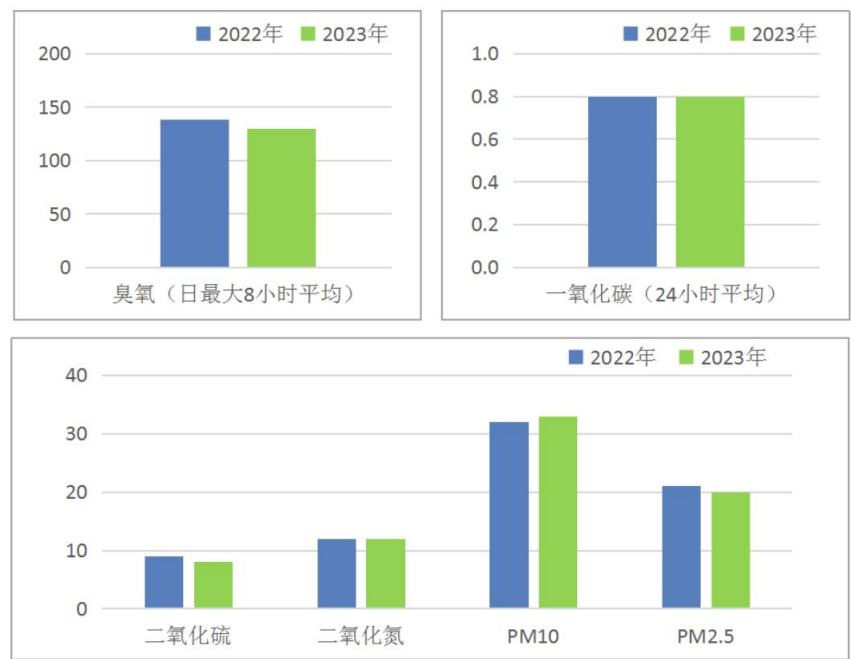
图 3-14 2023 年湛江市空气环境监测项目季评价对比图 (一氧化碳单位为 mg/m 3 、其他项目单位为 μg/m 3 )
