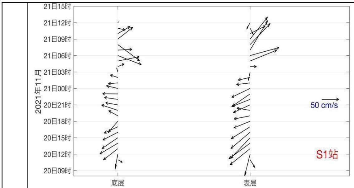
图 3-10a S1 站实测海流矢量图
